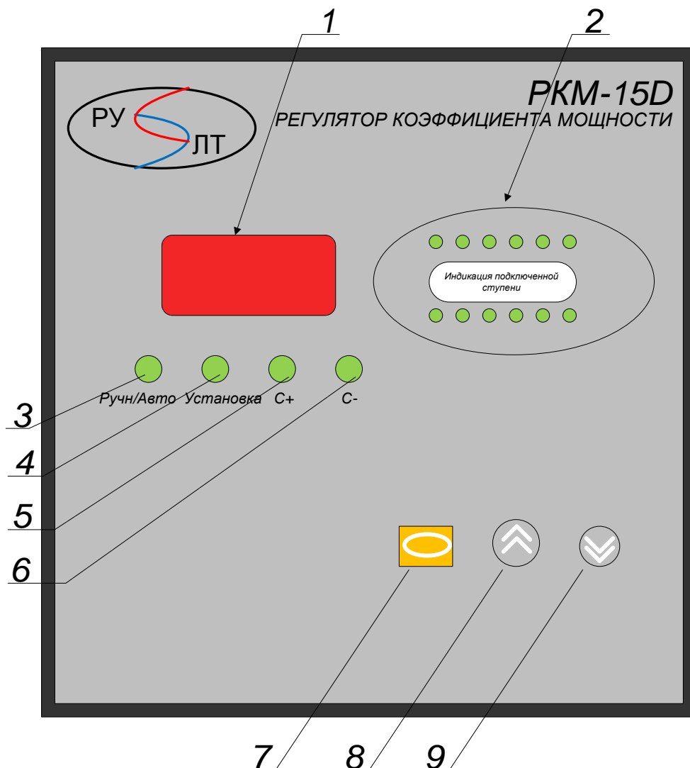
Рисунок. 1 Регулятор реактивной мощности
