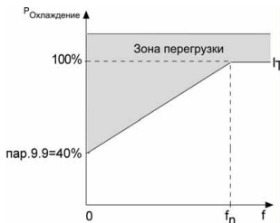
Рисунок 9.8: Эффективность охлаждения
